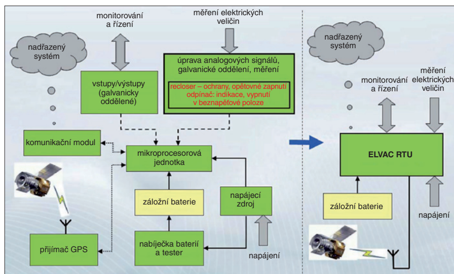
Obr. 1. Řešení tzv. all-in-one – všechny potřebné moduly jsou v jednom šasi
