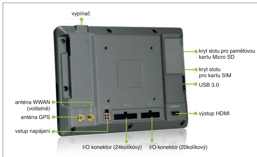
Obr. 2. Panelový počítač AFOCAR-08 A – pohled zezadu
