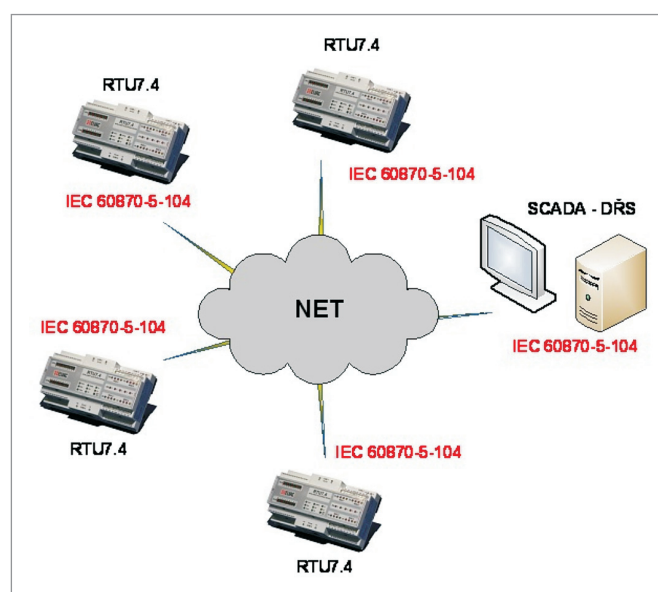
RTU7.4 pro dispečerské řízení
