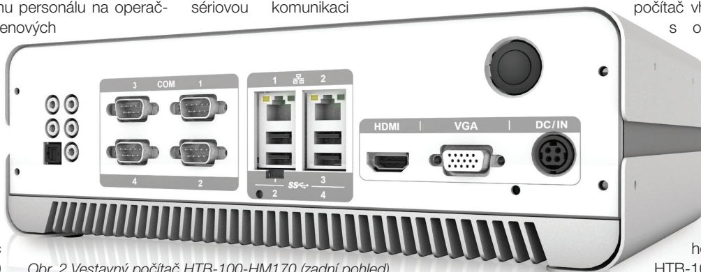
Obr. 2 Vestavný počítač HTB-100-HM170 (zadní pohled)
