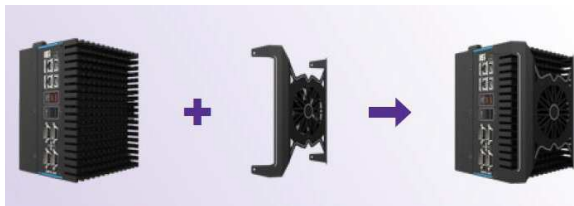
Volitelný externí ventilátor pro vytvoření aktivního proudění a odvodu tepla
