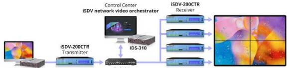
Snadné nasazení díky přepínání funkci Tx a Rx v jednom zařízení
