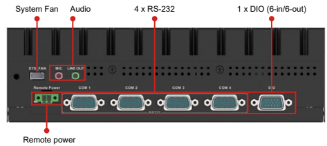
Pohled zezadu
